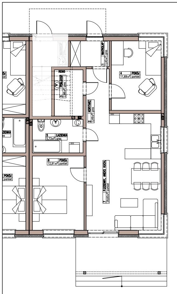
PARTER POWIERZCHNIA: 69,68m 2
